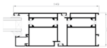
Dveře - řez
