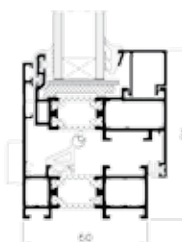
Okno otvíravé - řez
