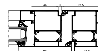
Dveře - řez
