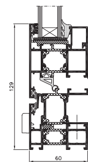
Okno otočné - řez
